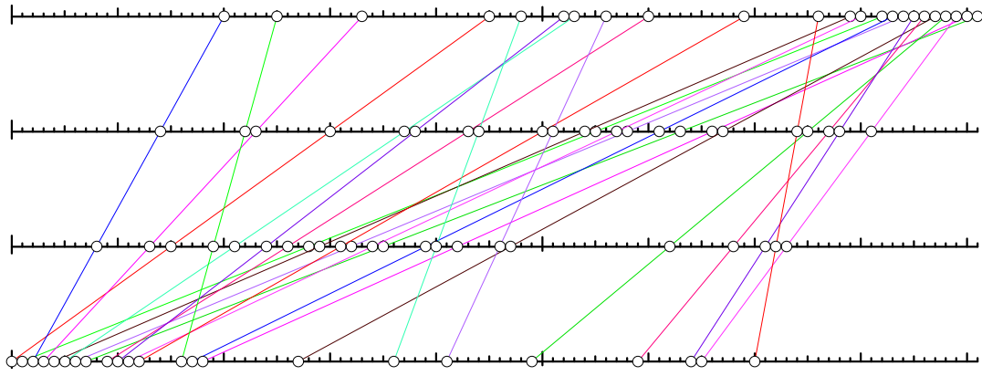
Représentation géométrique d'un pavage rythmique parfait n = 23, k = 4
